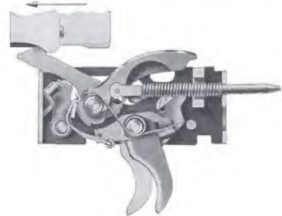
Fig: 30 Burst
